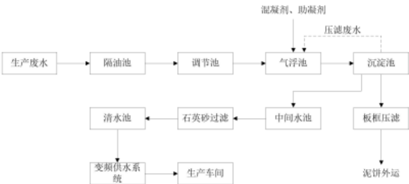
废水处理工艺流程图
